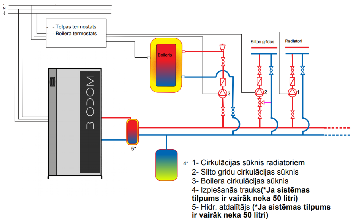
Pieslēguma shēma 2*
